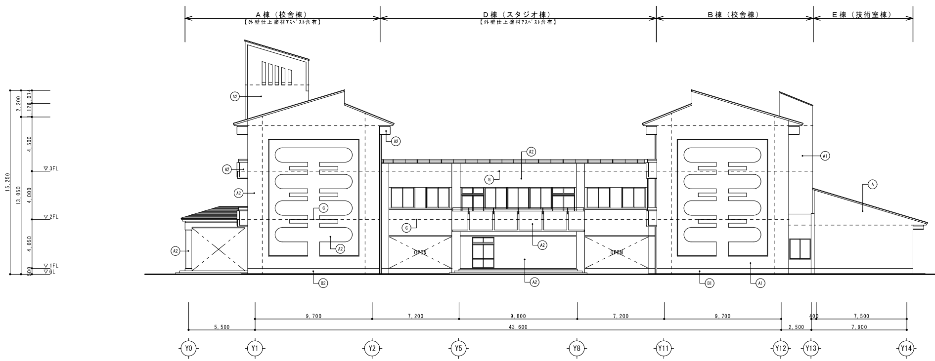
東 立面図 S=1:100 視点：グラウンド側から
