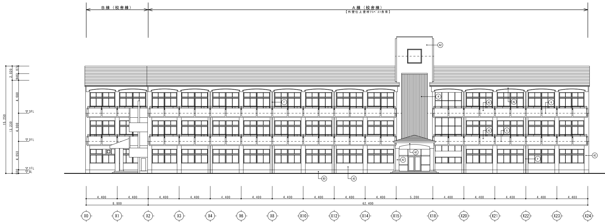
南 立面図 S=1:100 視点：校舎正面玄関側から
