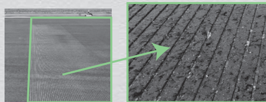
幅・深さ6mmの溝を3cm間隔で設置
