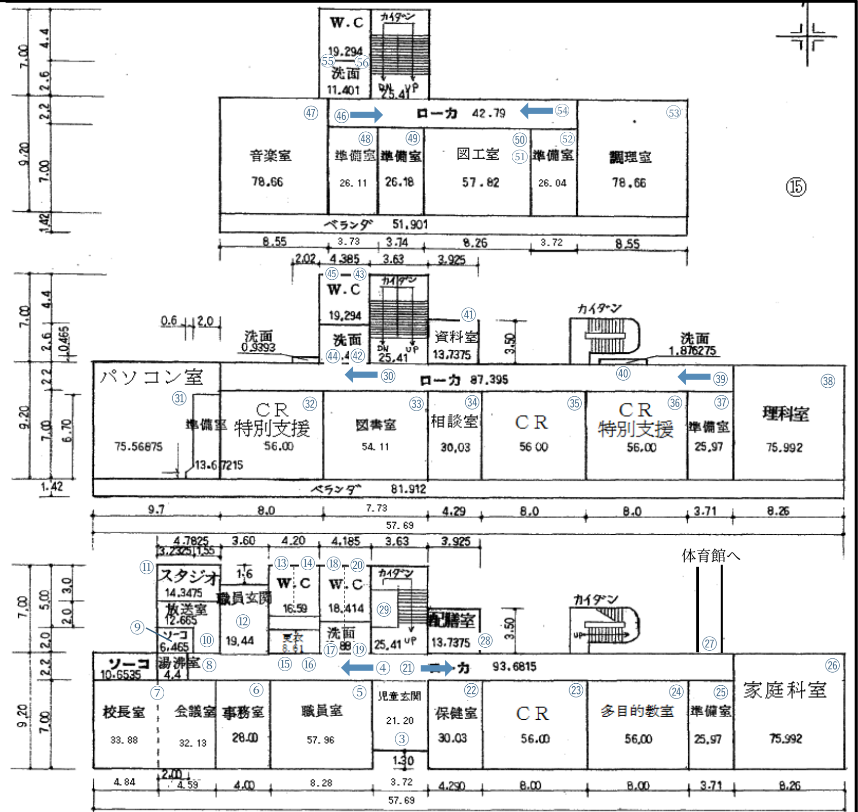
平面図
