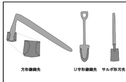
各種刃先図
